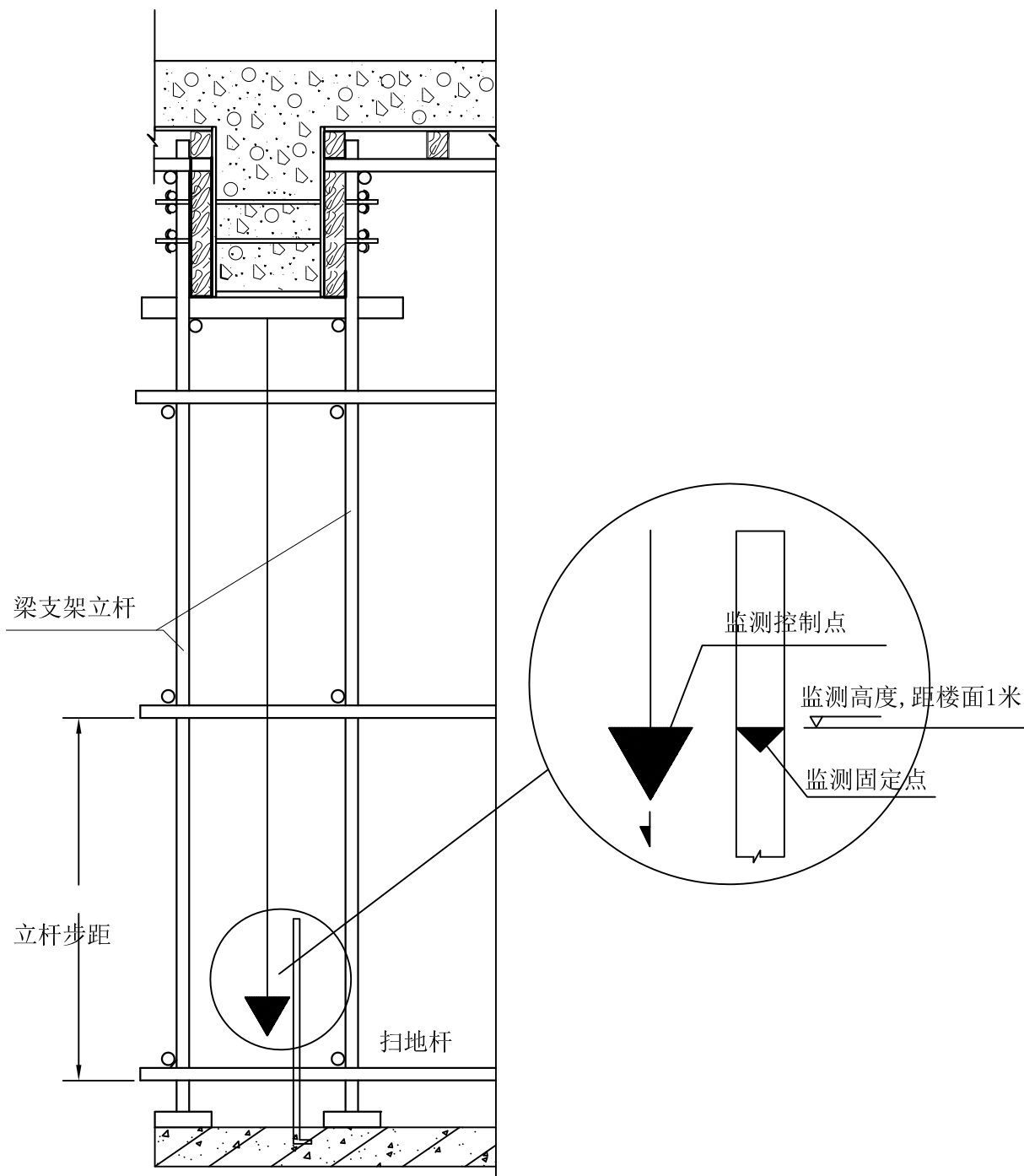
梁立杆横距 监测点示意图
