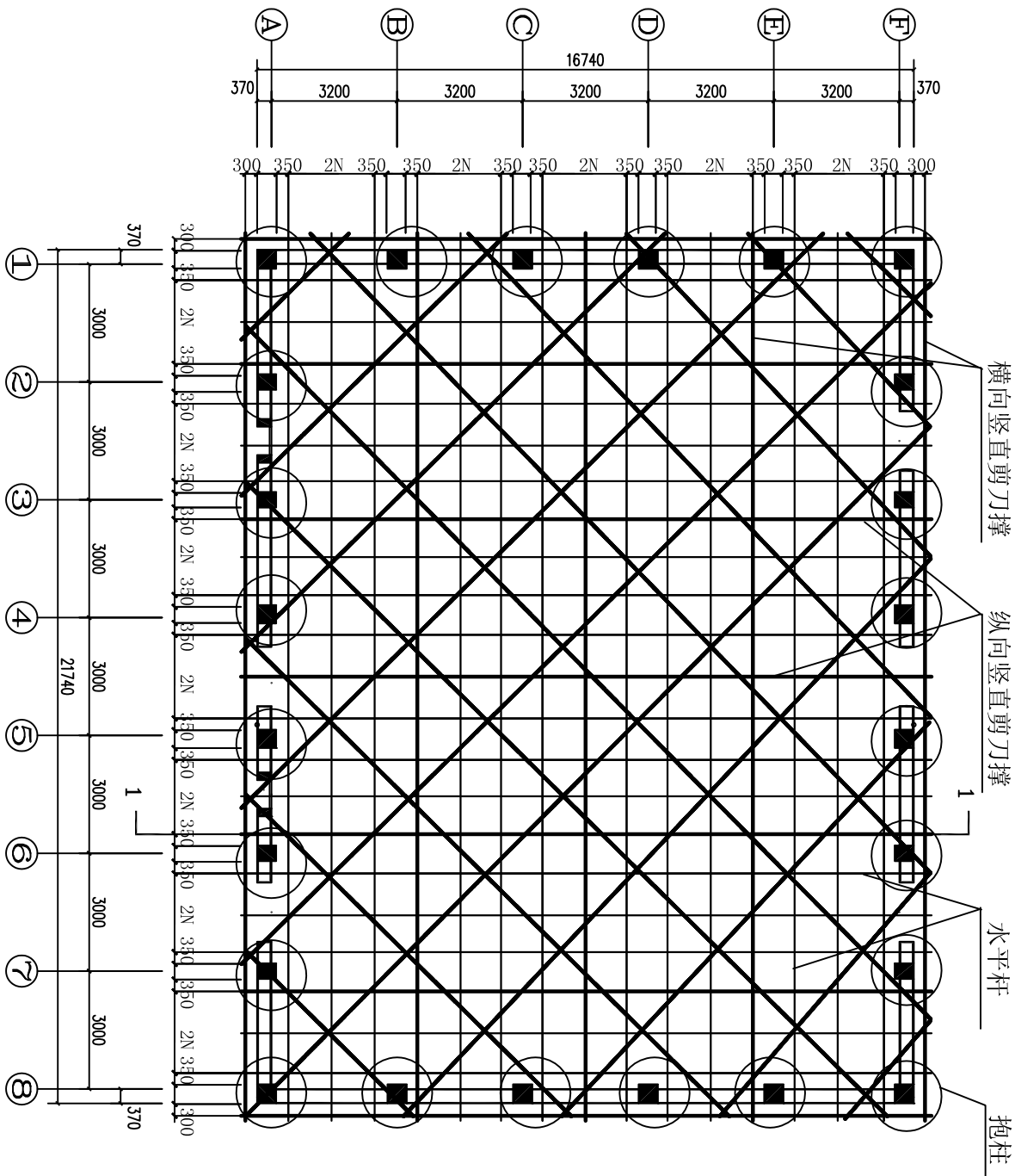
军供成品仓高大模板平面图
